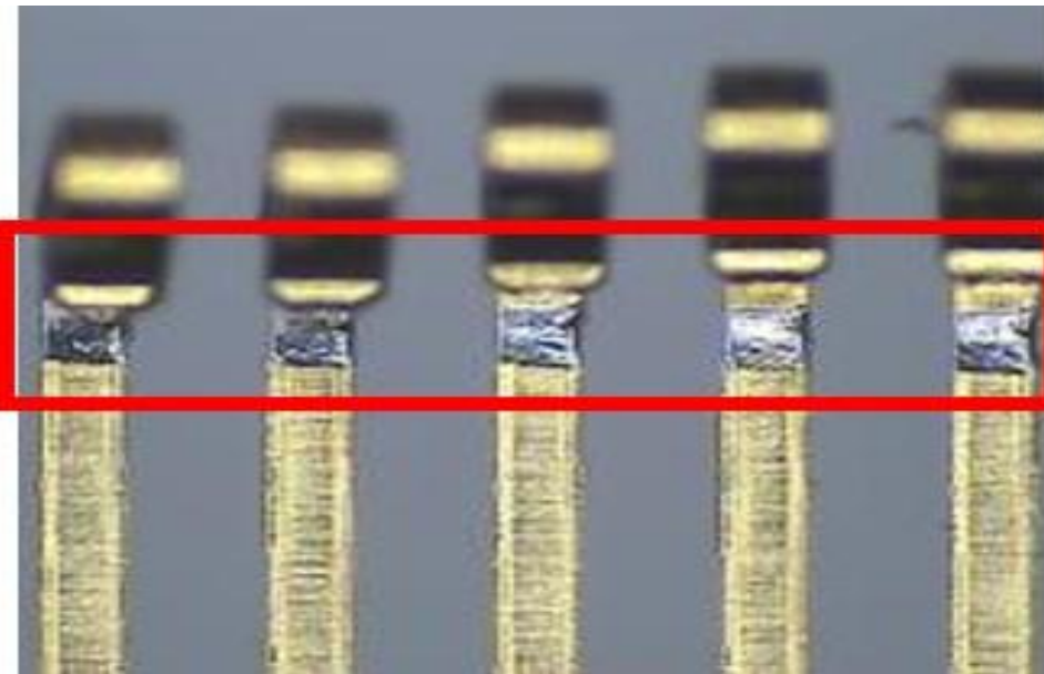
雷雕後 (雷雕尺寸0.12mm)
