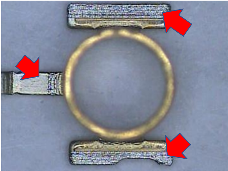
立體端子雷雕
